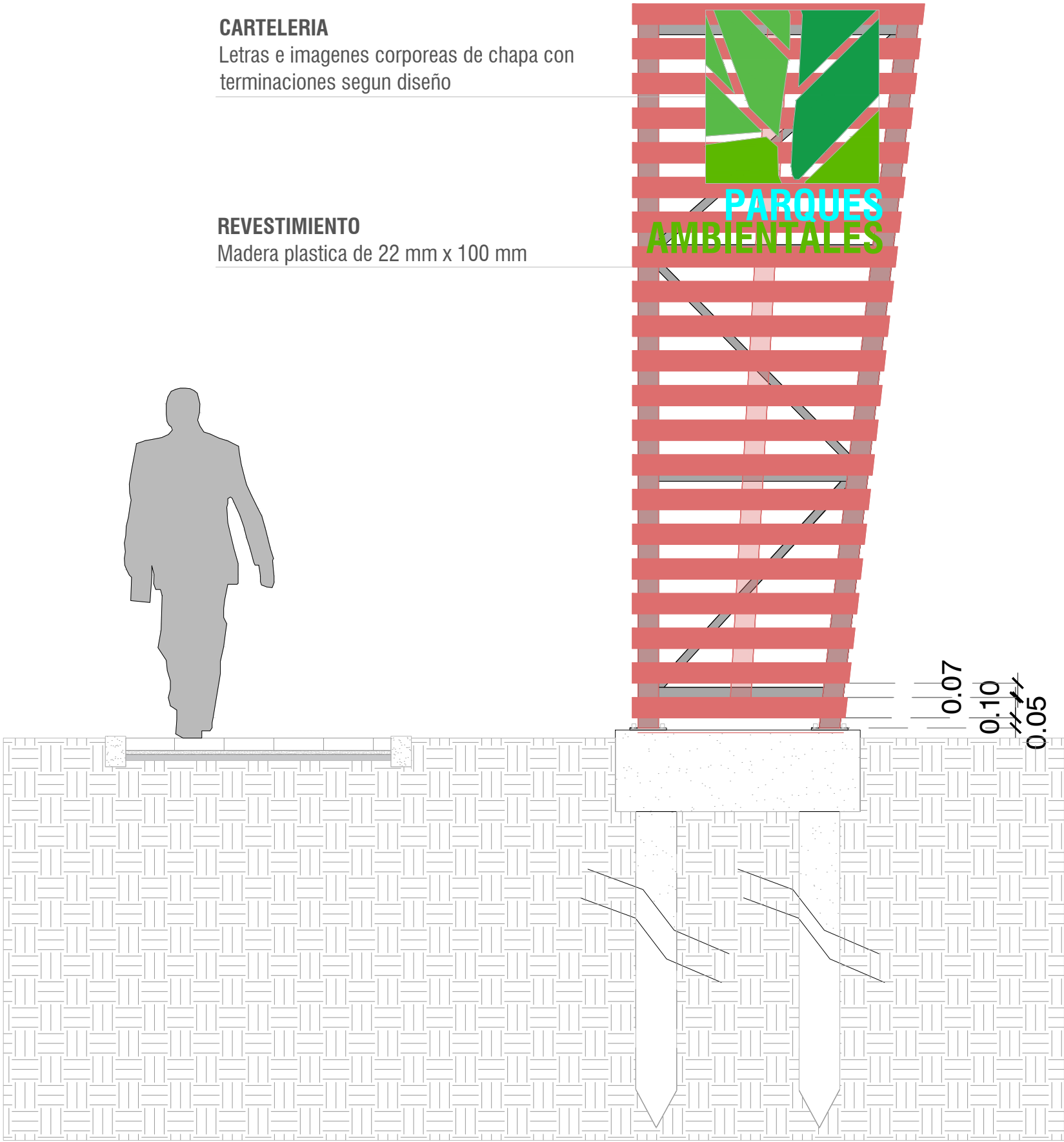
VISTA FRONTAL PLANO-2024-38923595-GDEBA-DPOATYB- CMAMGP
