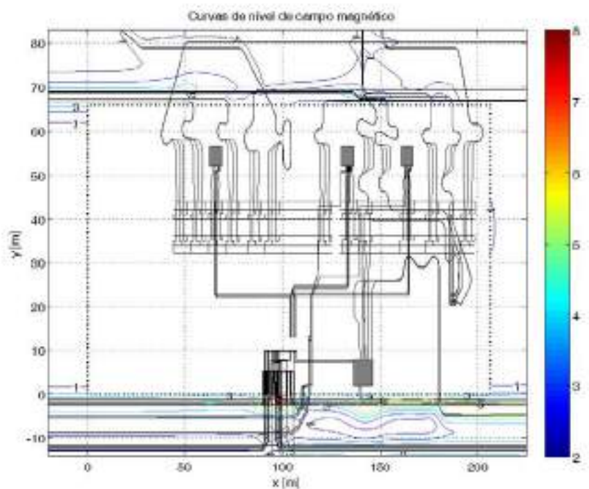
Figura AII- 4. Curvas de nivel de campo magnético en el borde perimetral de la SE, Caso 1.
