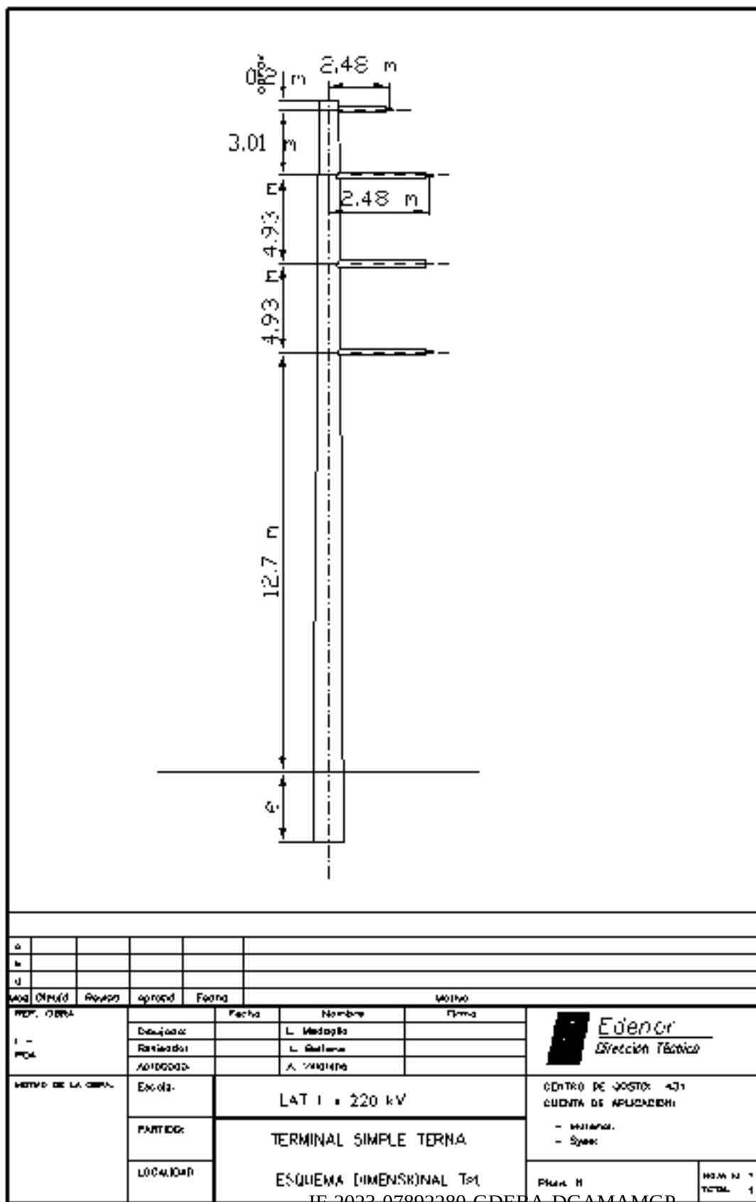
Figura AI-15. Corte línea aérea (220 kv).
