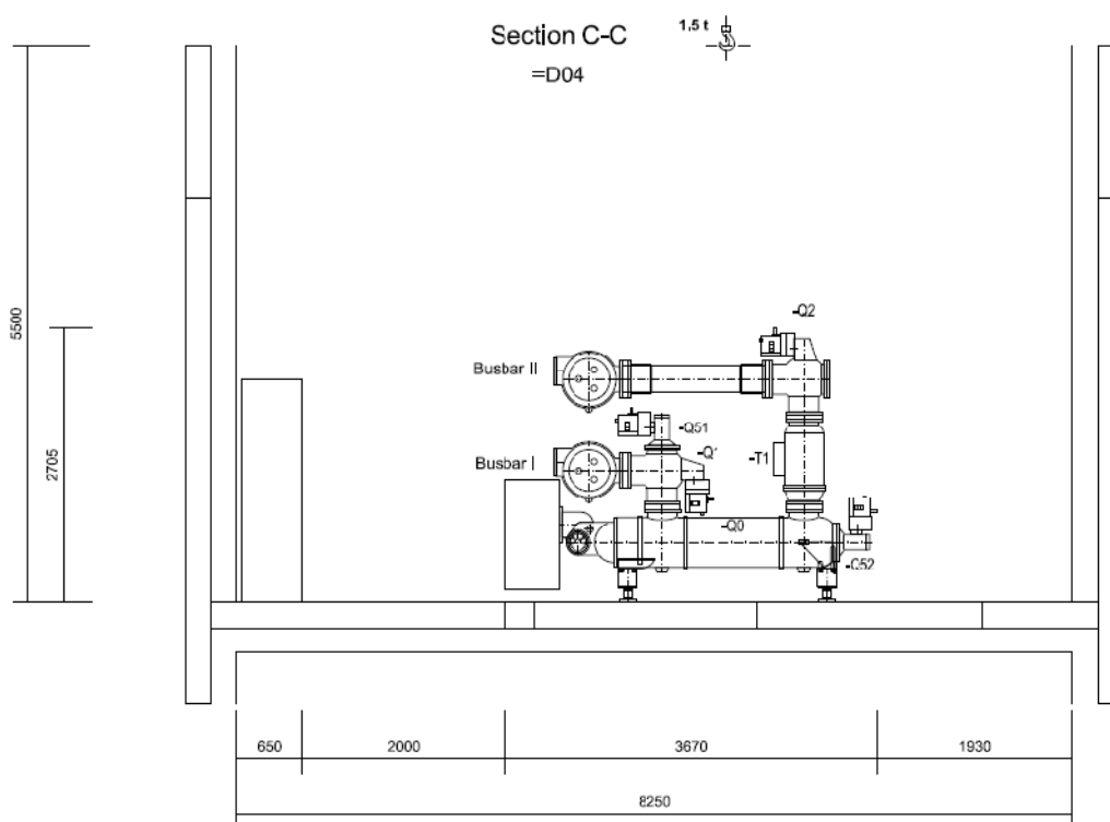
Figura AI- 7. Corte GIS en 220 kV.
