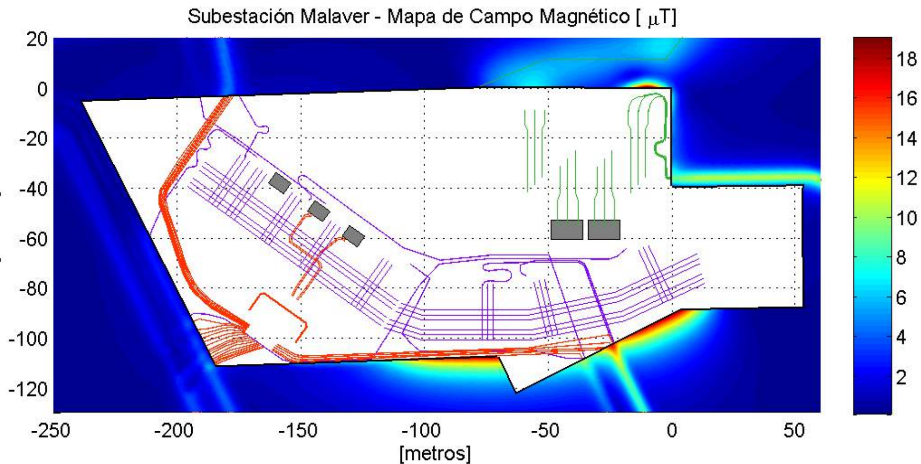
Figura 2. Caso I. Situación actual. Corrientes suministradas por EDENOR (balanceado).
