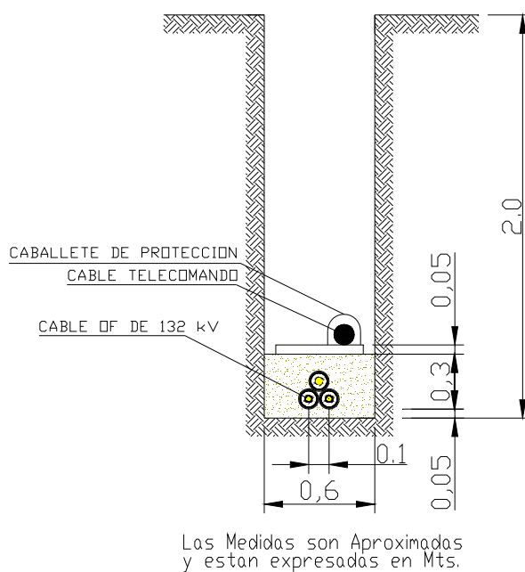
Figura AI- 20. Corte típico CS OF 1 x 132 kV.
