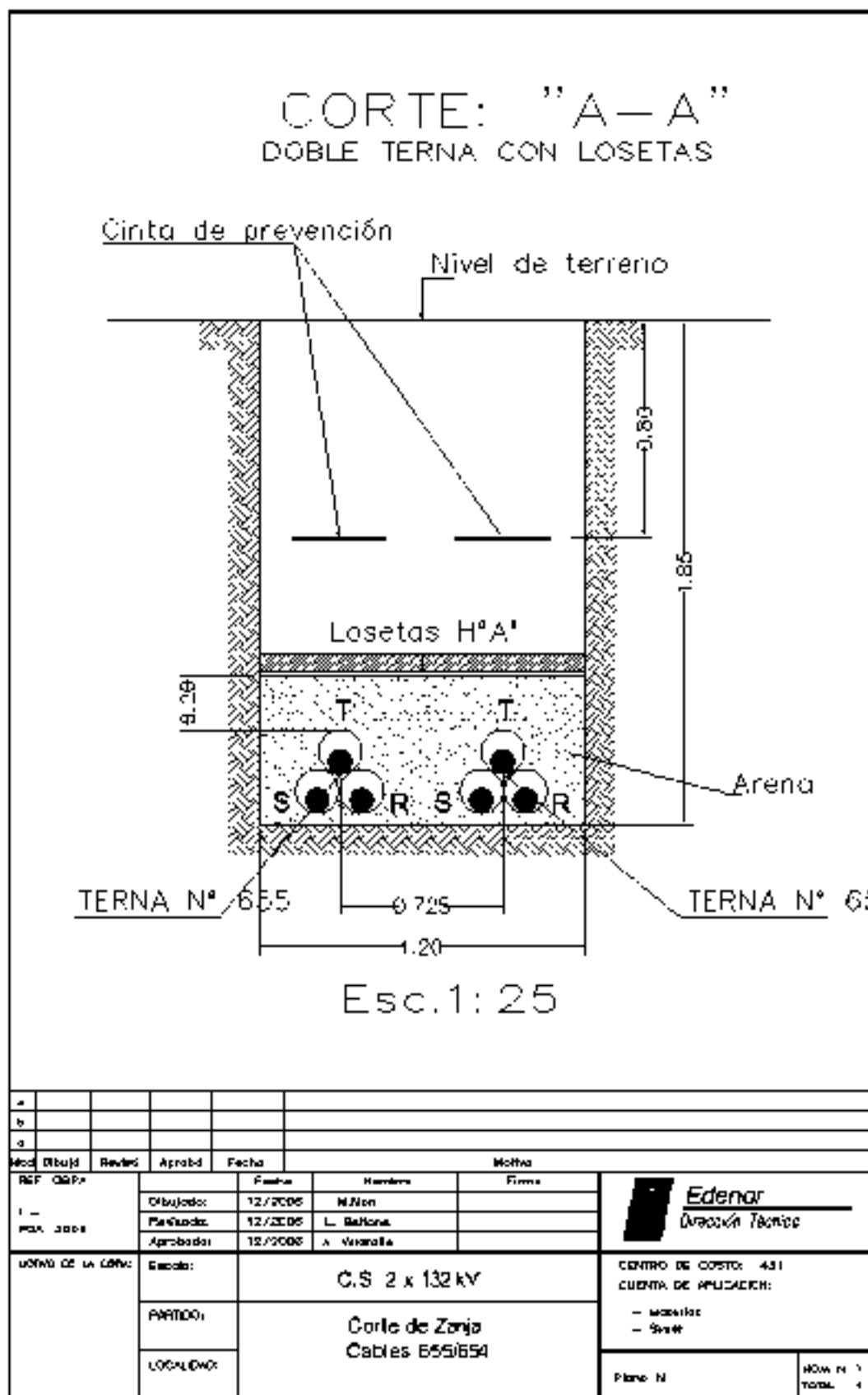
Figura AI-19. Corte cable 132 kV. Cables 655 – 656.
