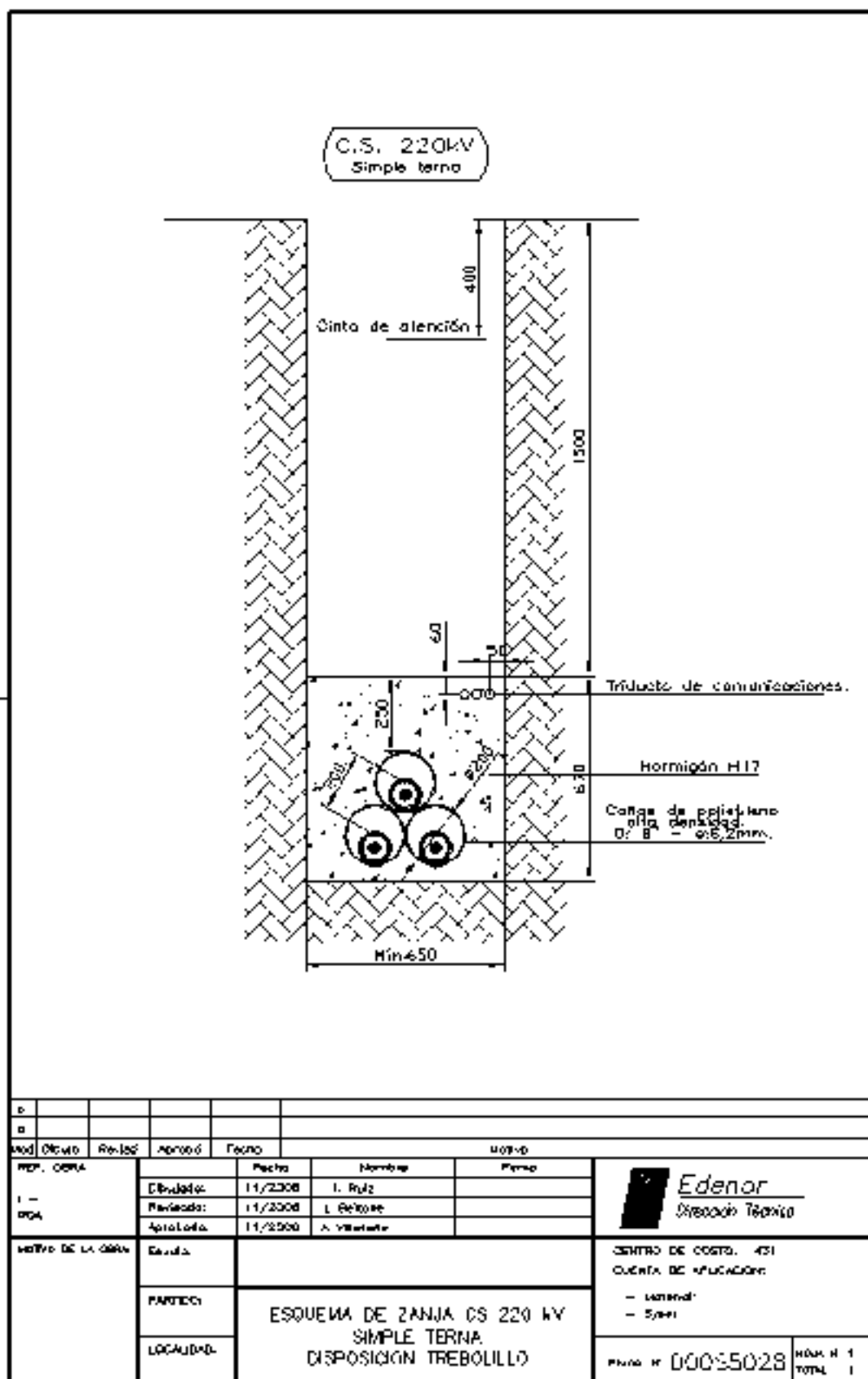
Figura AI-17. Corte cable 220 kV. Disposición tresbolillo.
