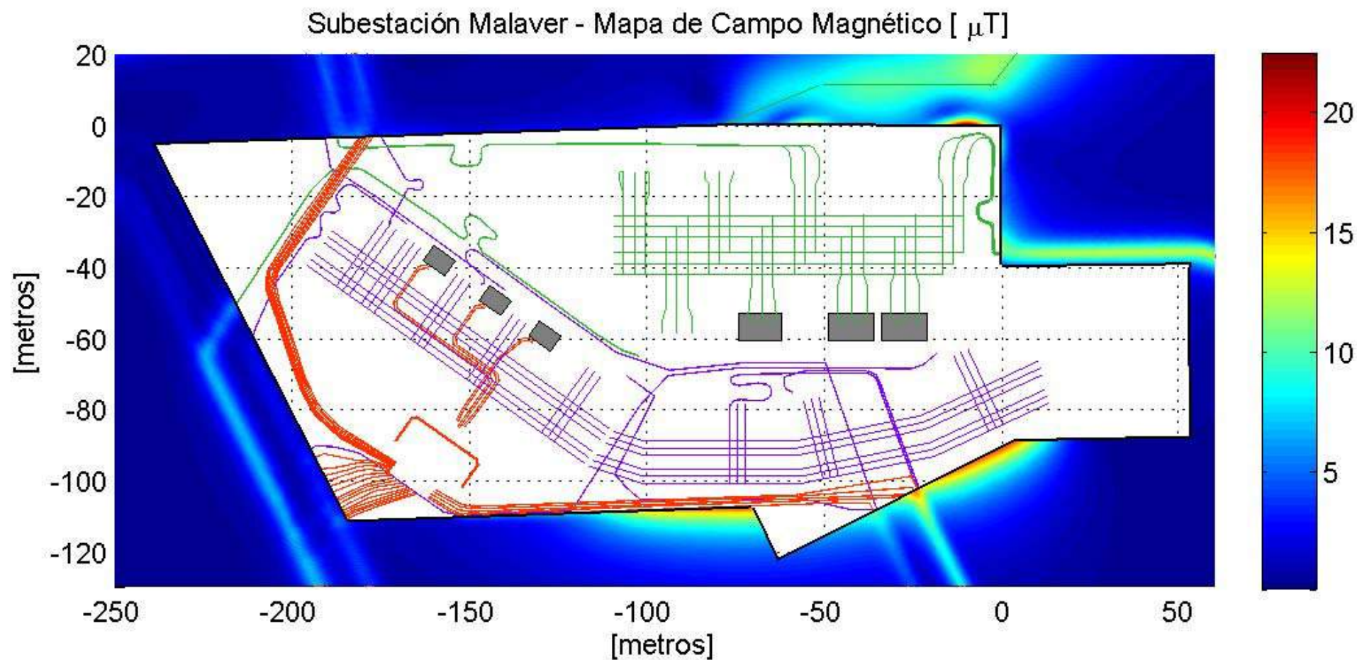
Figura 6. Caso V. Situación Futura. Corrientes suministradas por CAMMESA (balanceado).
