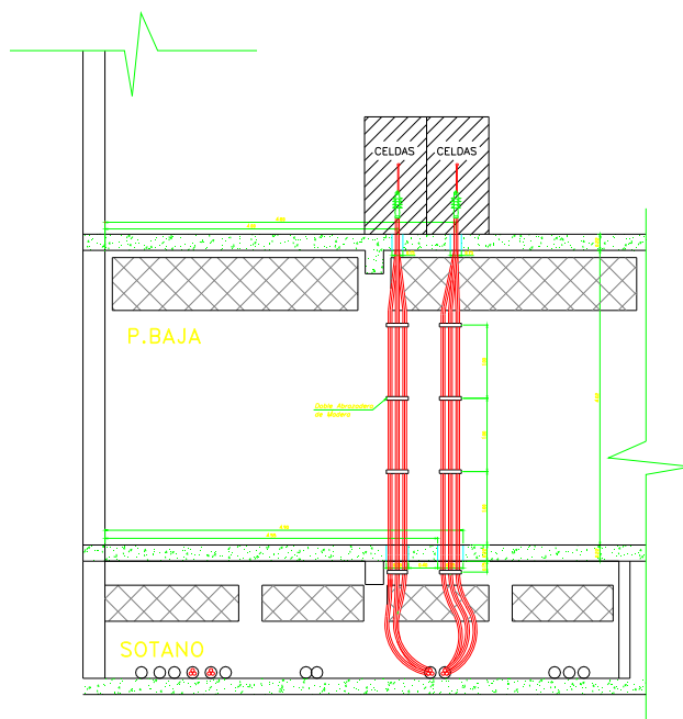
CORTE C-C ESC. 1:50
