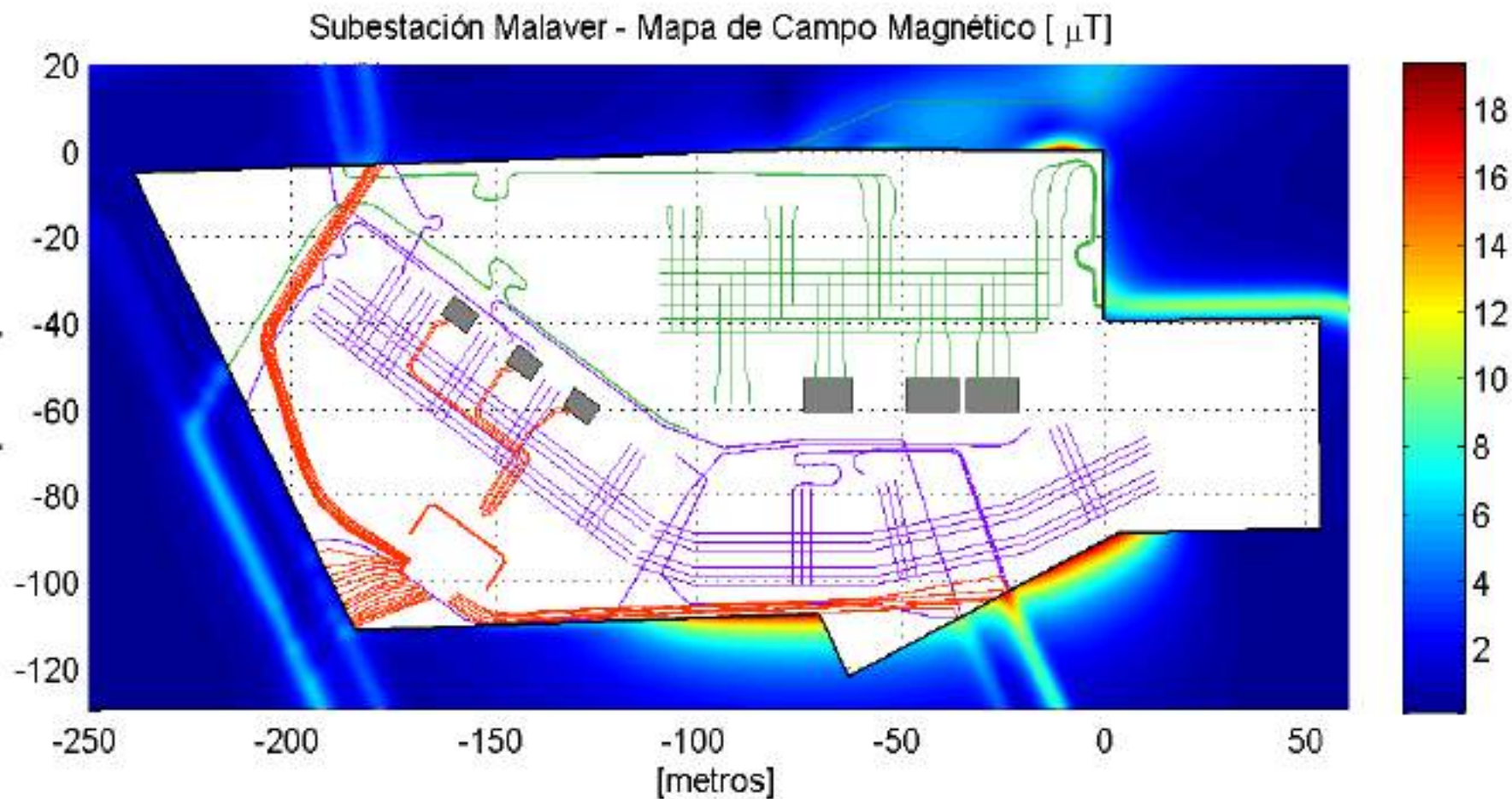
Figura 4. Caso III. Situación futura. Corrientes suministradas por EDENOR (balanceado).
