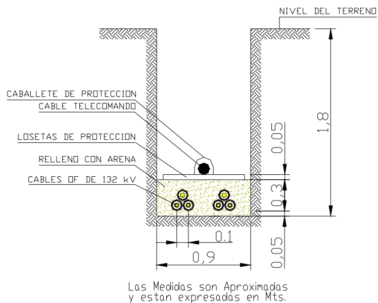
Figura AI- 19. Corte típico CS OF 2 x 132 kV.
