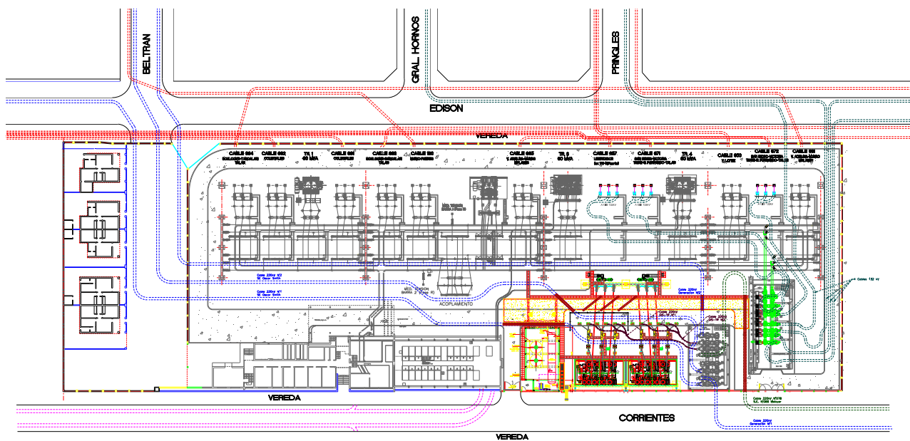
Figura AI- 3. Acometidas de alta tensión (Ampliación Etapa 2) Plano N° 078A5034
