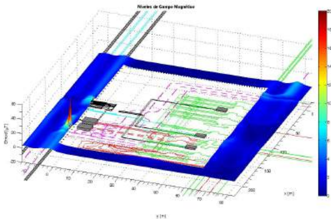
Figura 6. Niveles de Campo magnético, Caso 2.
