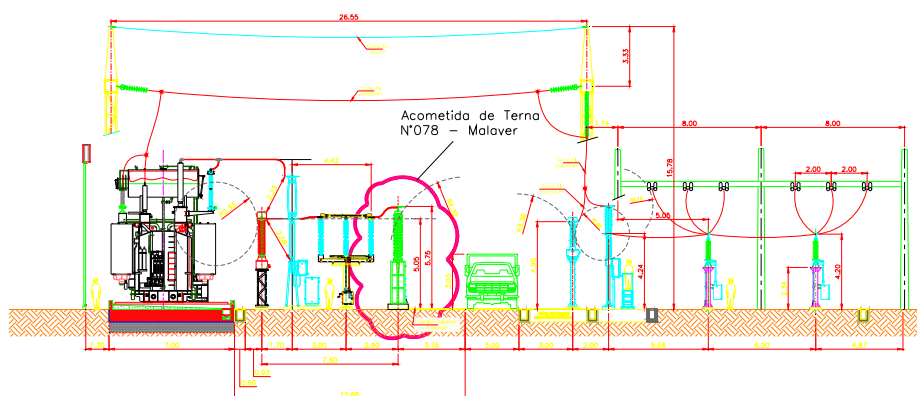
Figura A1- 4. Corte Campo de transformador 220 kV y barras en aire en 132 kV.
