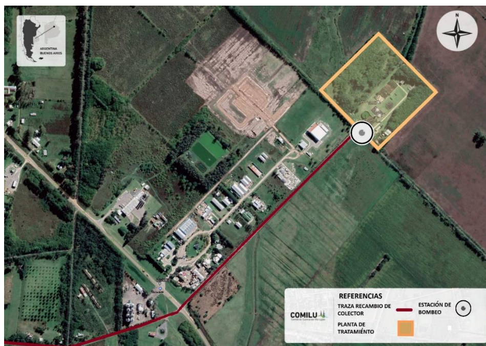
Figura 3- Estación de Bombeo en Planta de tratamiento.
