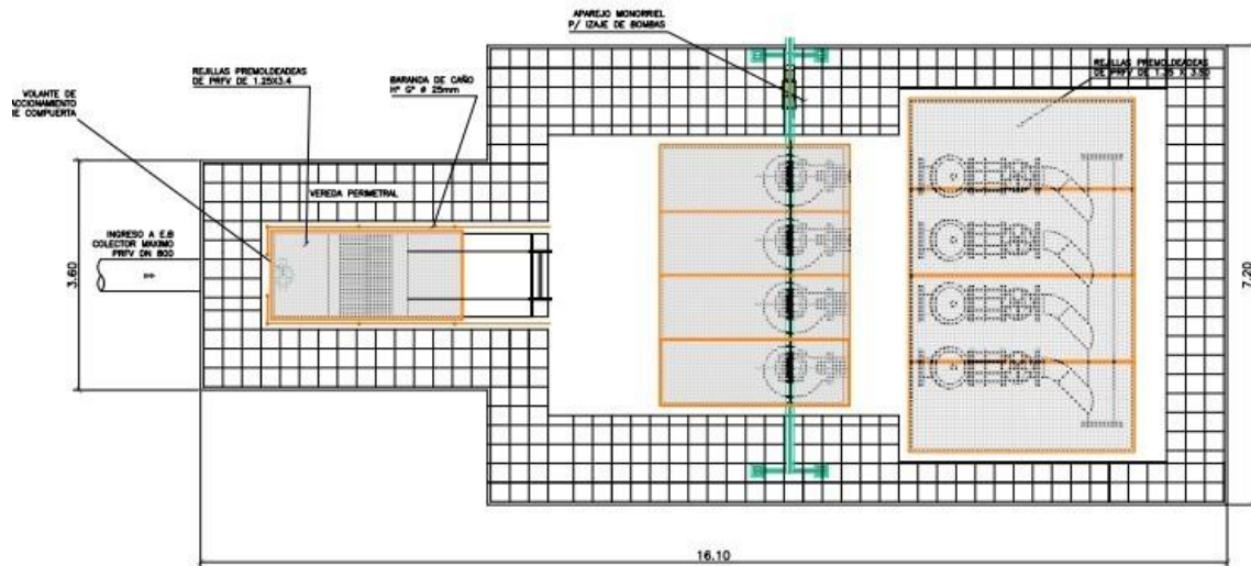
Figura 4- Planta de Estación de Bombeo
