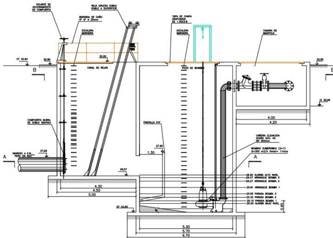
Figura 5- Corte Longitudinal de la Estación de Bombeo
