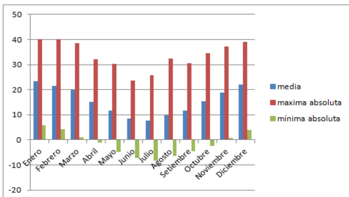
Figura 15: Valores promedio mensuales y anuales; valores máximos absolutos de temperatura, Estación Bahía Blanca Aero, período 1991-2000
