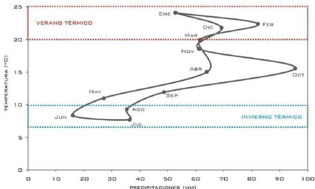
Figura 14: Climograma. Estación Bahía Blanca Aero (2001-2010)
