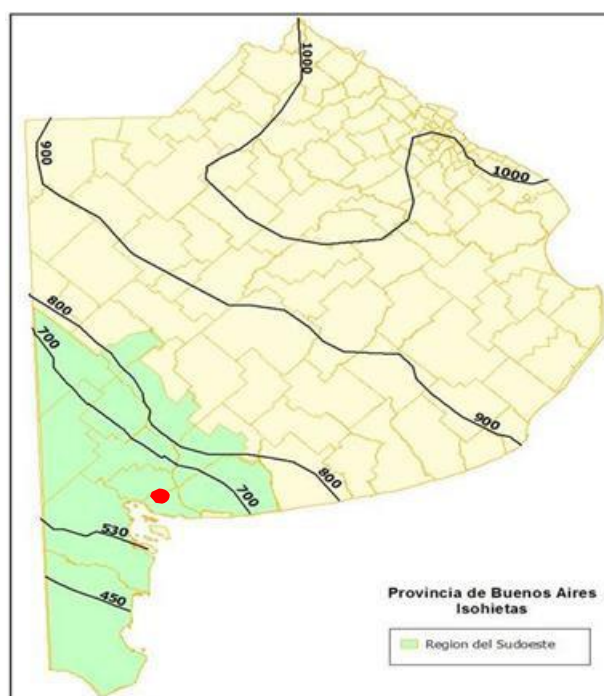
Figura 12: Isohietas de la Provincia de Buenos Aires y de la Región Sudoeste Bonaerense
