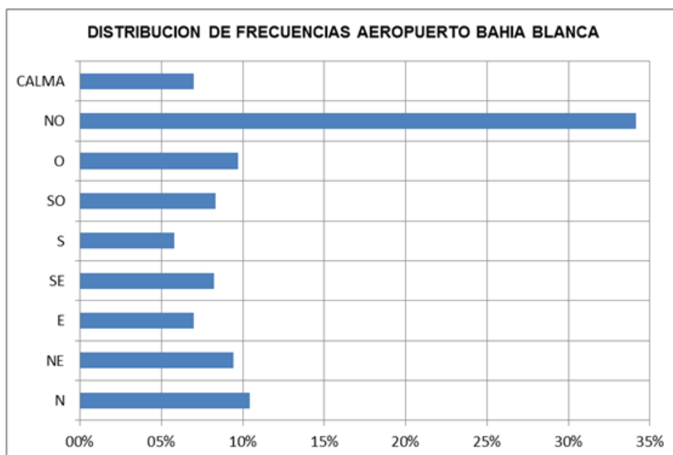
Figura 18: Frecuencia devientos
