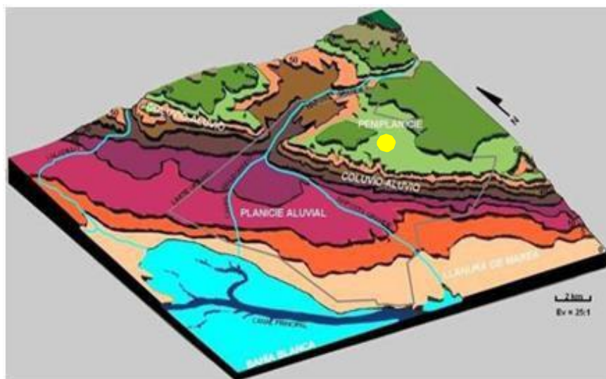
Figura 24: Diagrama topográfico
