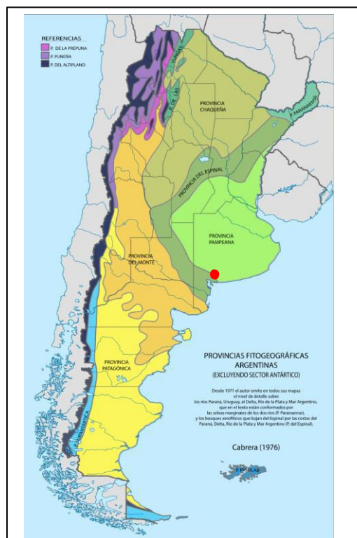
Figura 28: Regiones Fitogeográficas según Cabrera (1976)
