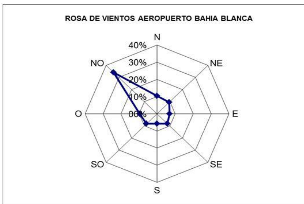
Figura 20: Rosa de vientos con las frecuencias medias anuales según dirección Fuente: Elaboración propia a partir de datos del Servicio Meteorológico Nacional
