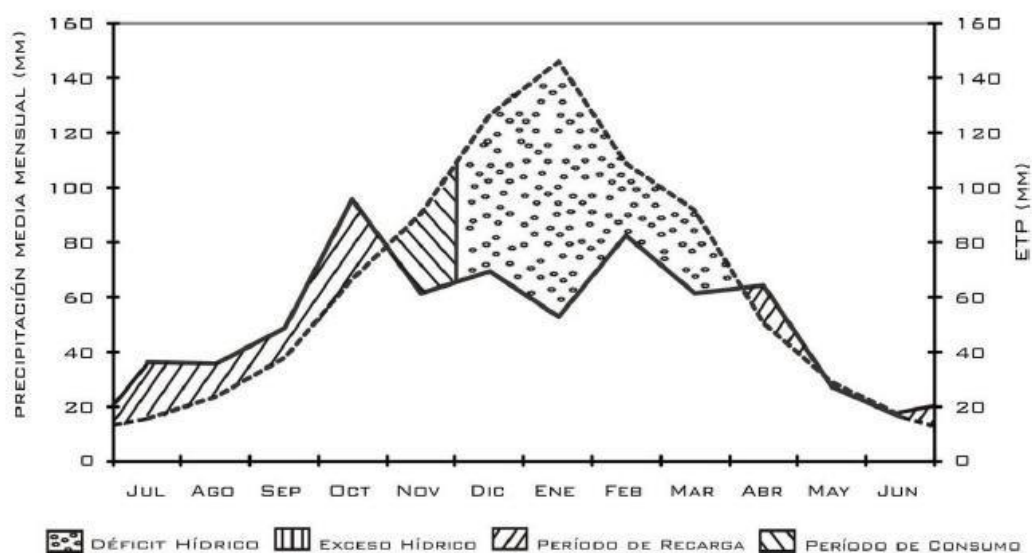
Figura 22: Balance Hídrico según datos de la Est. Bahía Blanca Aero (2001-2010)
