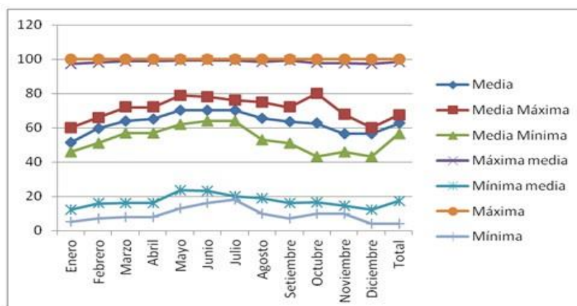
Figura 17: Valores promedio mensuales de humedad relativa, máximos y mínimos mensuales, y medias. Estación Bahía Blanca Aero. Periodo 2001 - 2010
