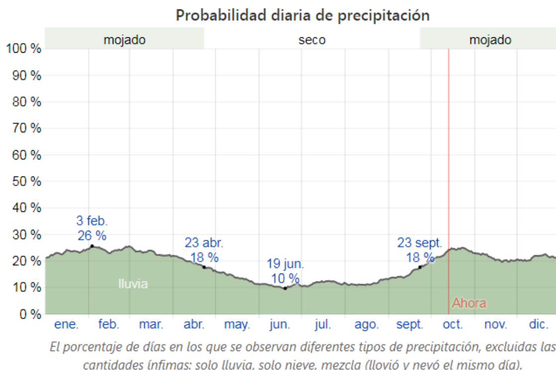
Figura 16: Probabilidad diaria de precipitación
