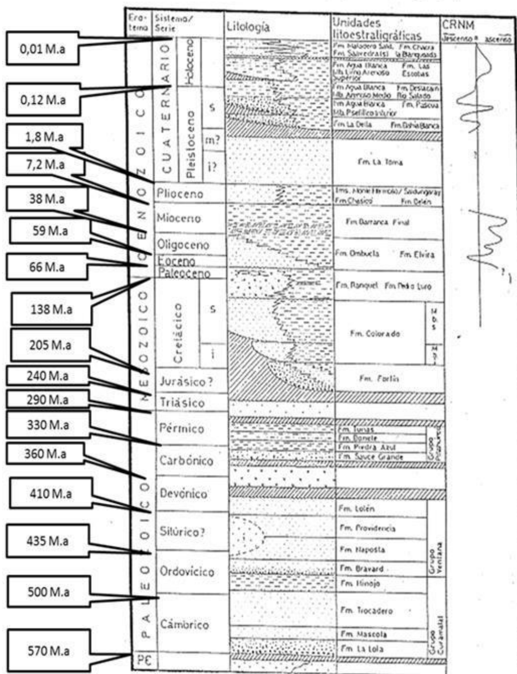
Figura 23: Cuadro estratigráfico. Quattrocchio - Zavala
