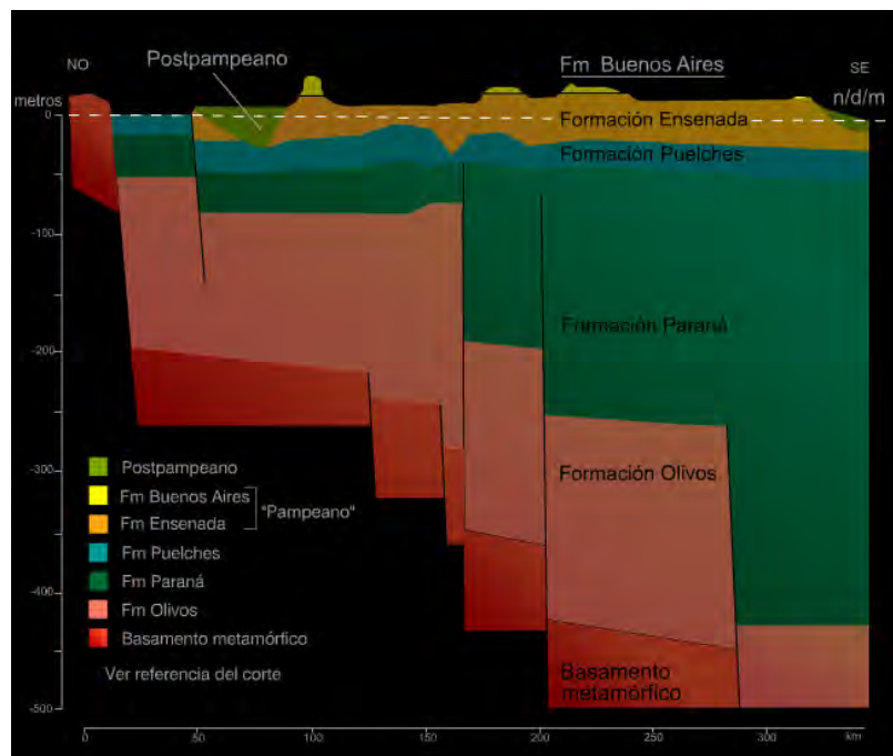
Figura 7: Esquema de corte estratigráfico suelo – subsuelo
