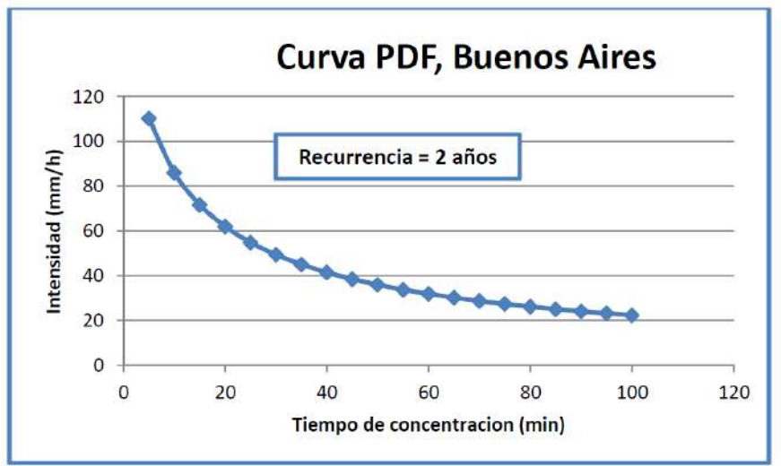
Figura 1. Curva de Precipitación, Partido de San Miguel. Obras Públicas Municipalidad de San Miguel
