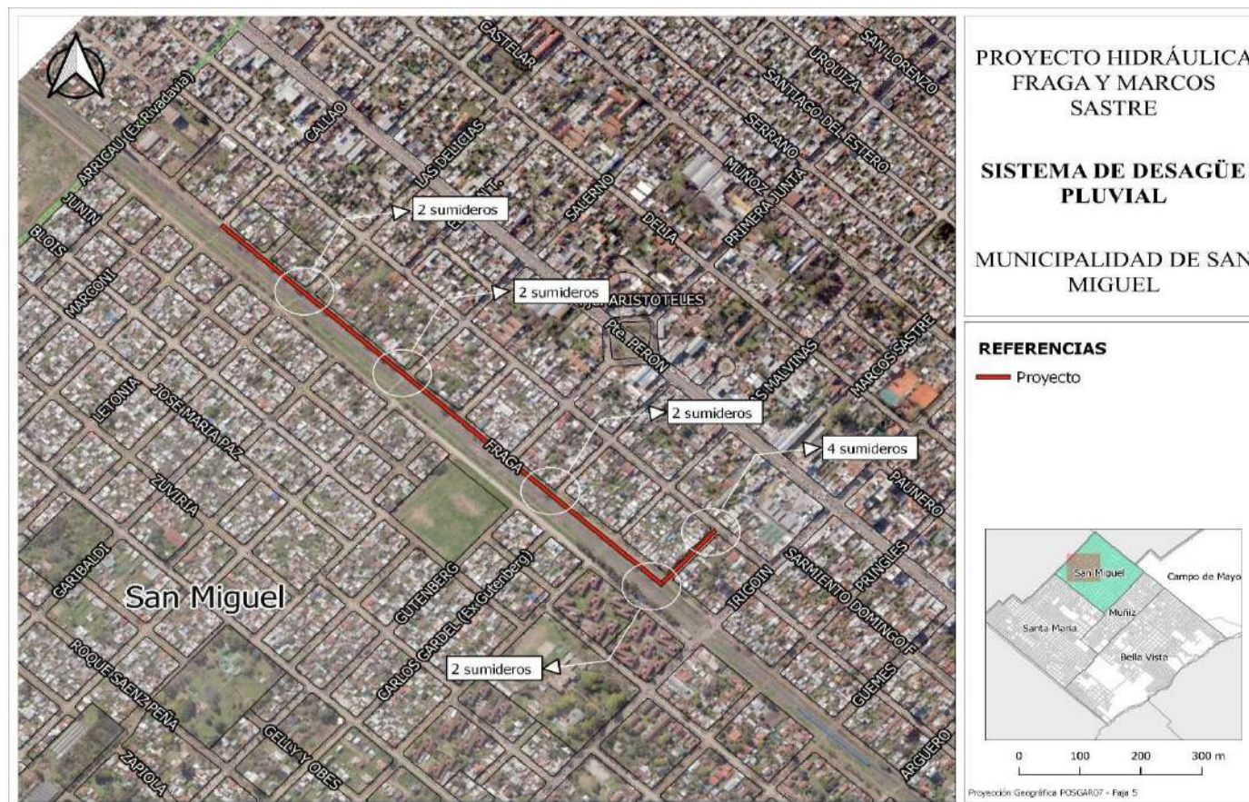
Figura 4. Proyecto Hidráulica Fraga y Marcos Sastre, Partido de San Miguel.
