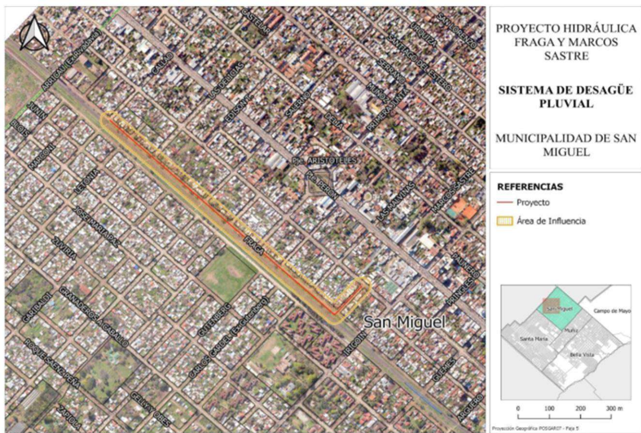
Figura 1. Esquema del área del Proyecto Hidráulica Fraga y Marcos Sastre - San Miguel. Fuente: GIS - Geomática - IDE - Municipalidad de San Miguel, Buenos Aires, Argentina.
