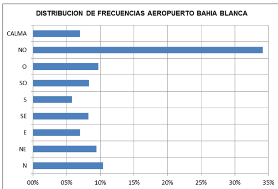
Figura 14: Frecuencia devientos
