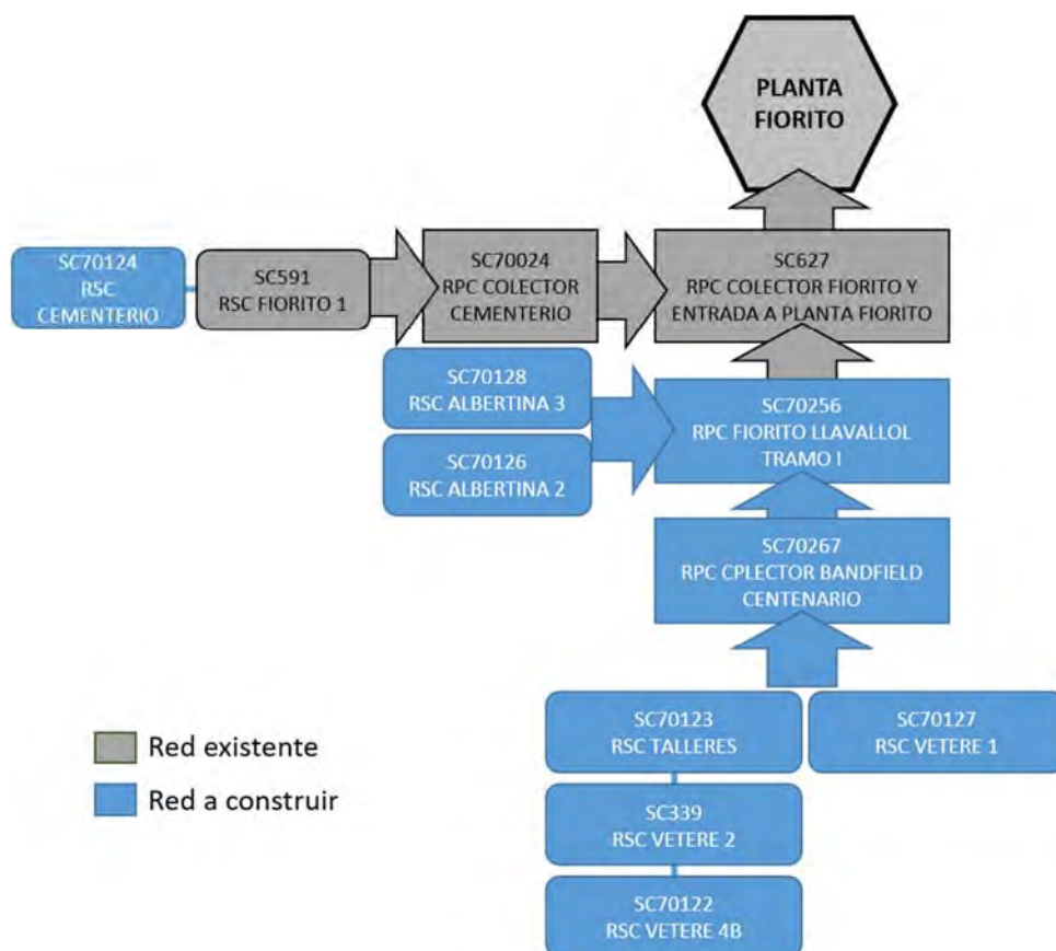
Figura 3: Esquema de vuelco del sistema
