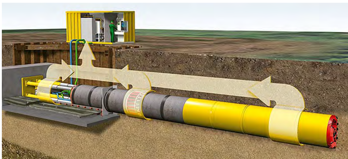
Figura 7: Esquema metodología constructiva pipe – jacking
