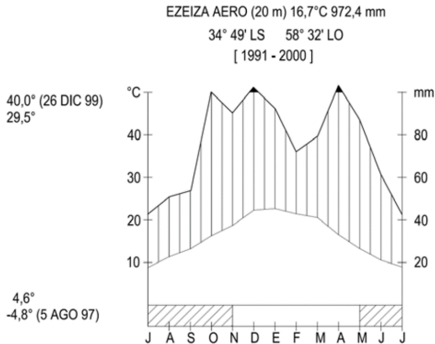
Figura 16: Climatograma período 1991–2000
