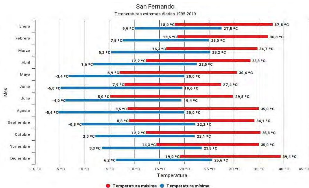
Figura 17: Temperaturas (°C) extremas extrema diarias. Est. Met. San Fernando Aero, período 1995-2019.
