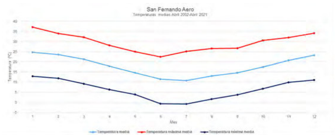
Figura 14: Temperaturas medias de la Est. Met. San Fernando Aero, período abril 2002-abril 2021.
