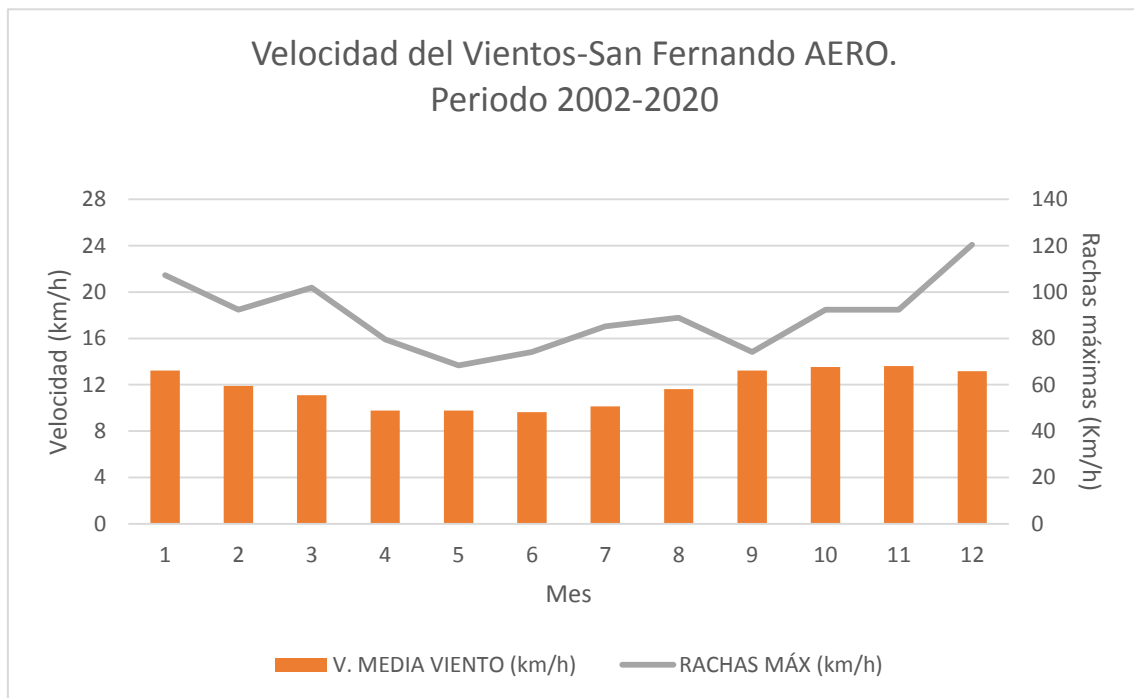
Figura 19: mensuales observados en Est. Met. San Fernando Aero, período 2002-2020. Fuente: https://www.meteored.com.ar
