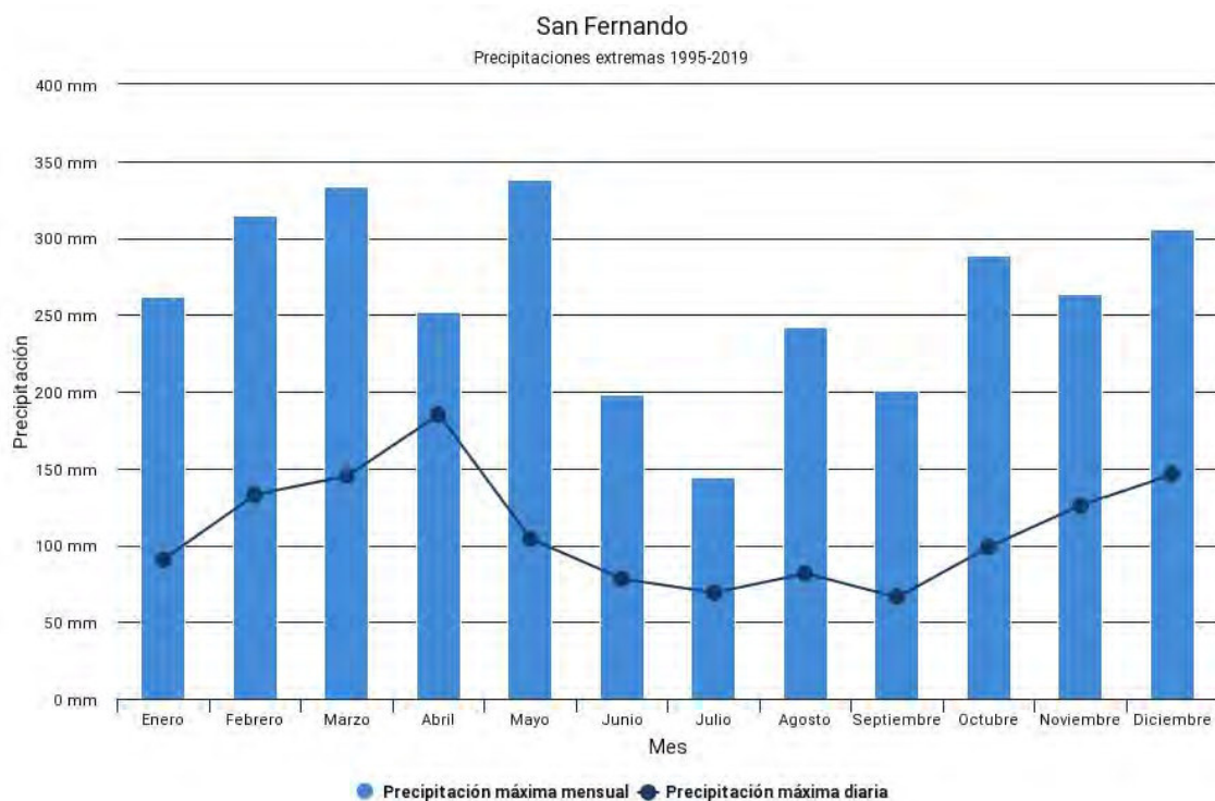
Figura 16: Precipitaciones extremas de San Fernando Aero, período 1995-2019. Fuente: www.smn.gob.ar/estadisticas .
