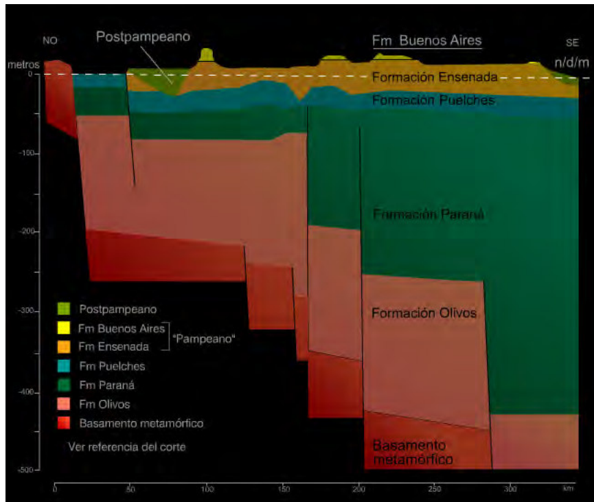
Figura 8: Esquema de corte estratigráfico suelo – subsuelo
