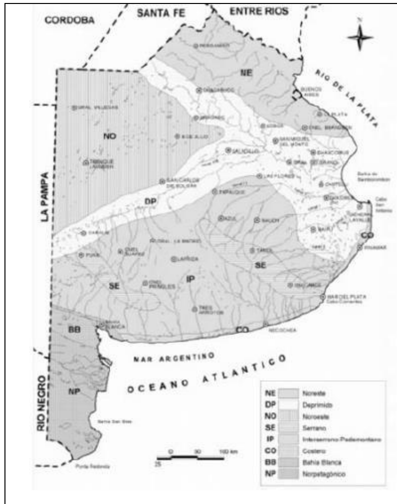
Figura 10: Regiones hidrogeológicas de la Provincia de Buenos Aires
