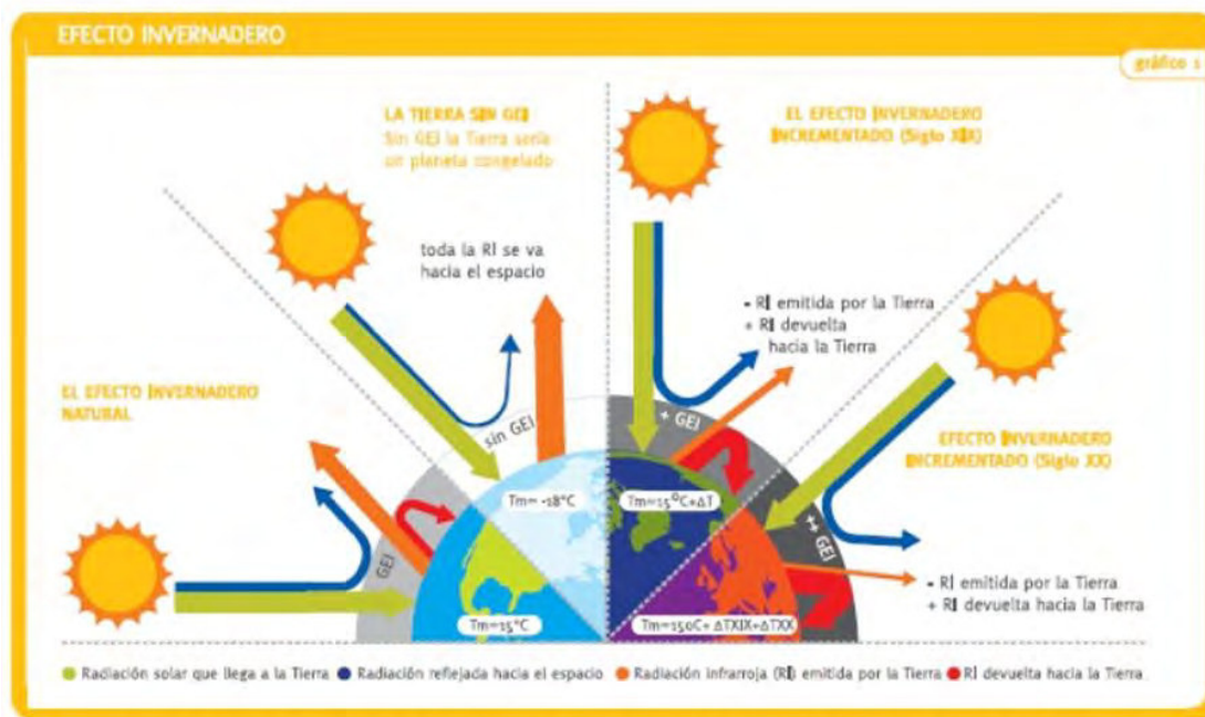
Figura 20: Diferentes escenarios posibles del efecto invernadero
