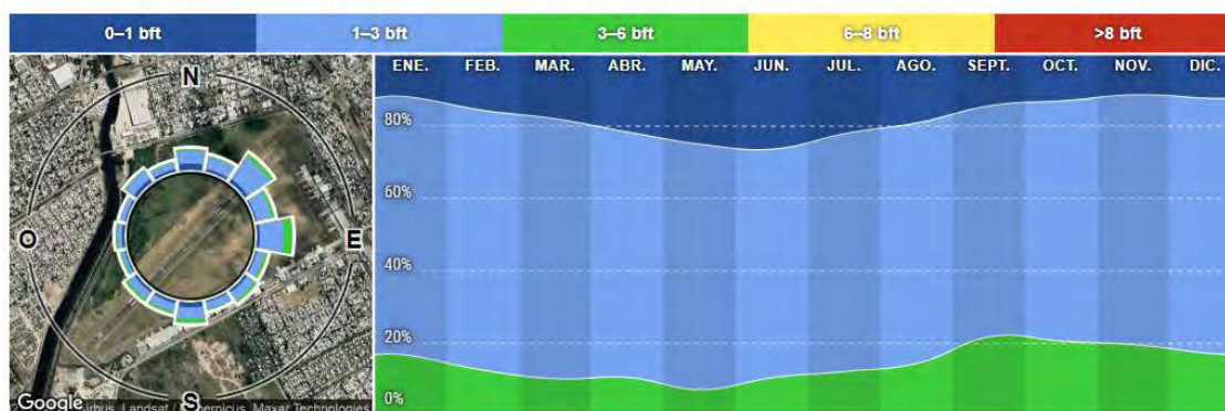
Figura 18: Estadísticas de Vientos en Est. Mat. San Fernando Aero, periodo 10/2008 - 03/2021. Estadísticas basadas en observaciones diarias. Dirección viento dominante, Distribución de dirección y fuerza del viento (% de tiempo, escala BFT 21 ).
