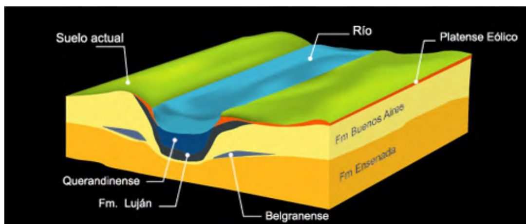
Figura 9: Esquema de formaciones pospampeana y pampeana
