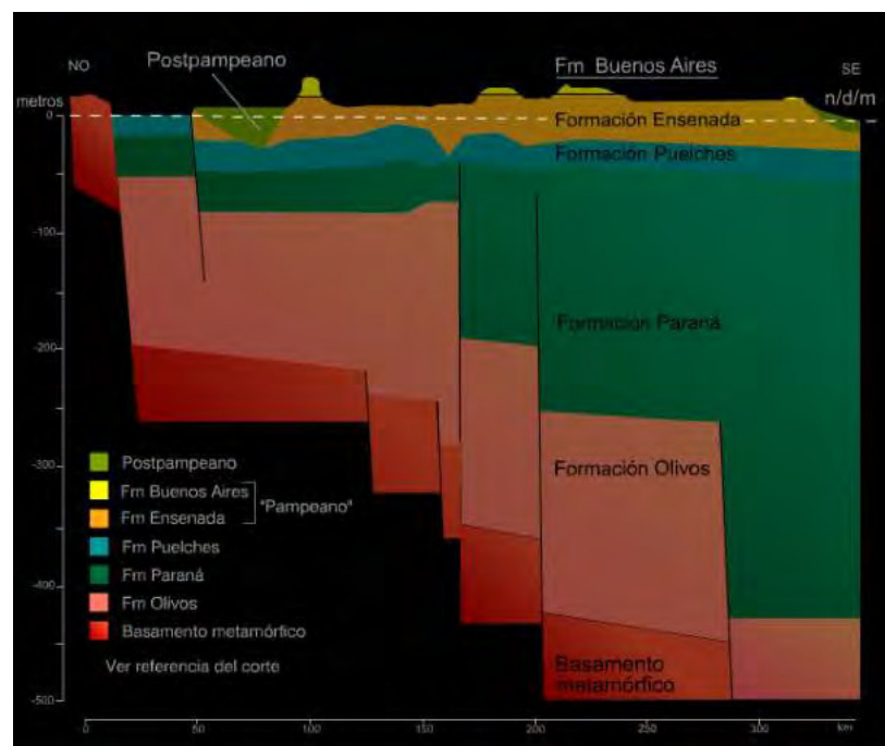
Figura 6: Esquema de corte estratigráfico suelo – subsuelo
