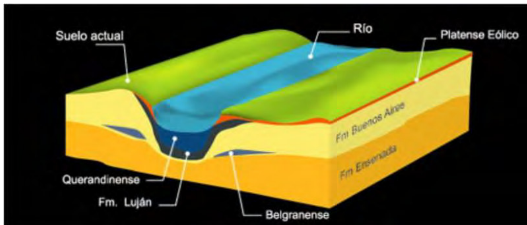
Figura 7: Esquema de formaciones pospampeana y pampeana
