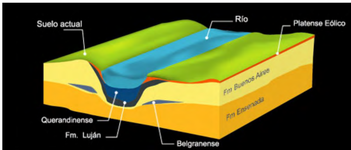
Figura 7: Esquema de formaciones pospampeana y pampeana
