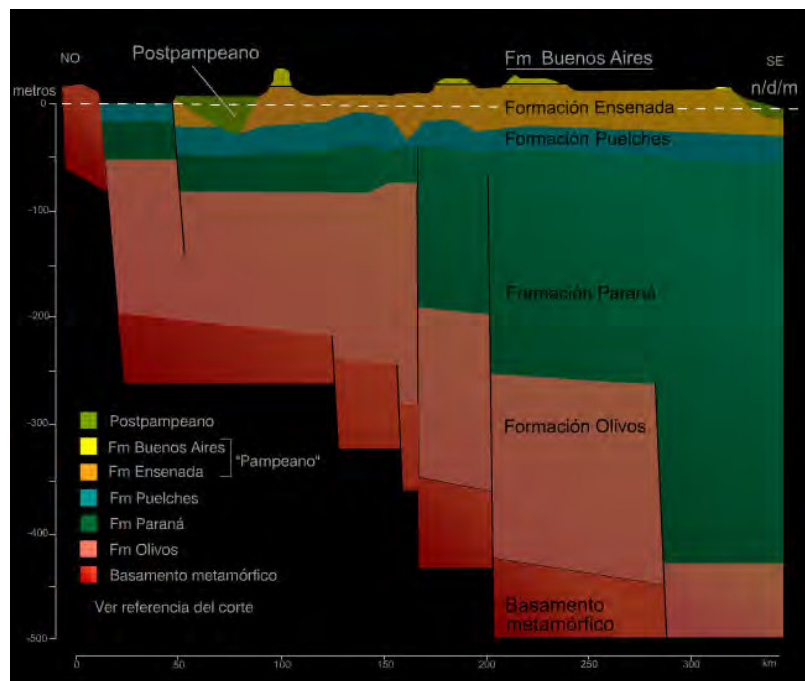
Figura 5: Esquema de corte estratigráfico suelo – subsuelo
