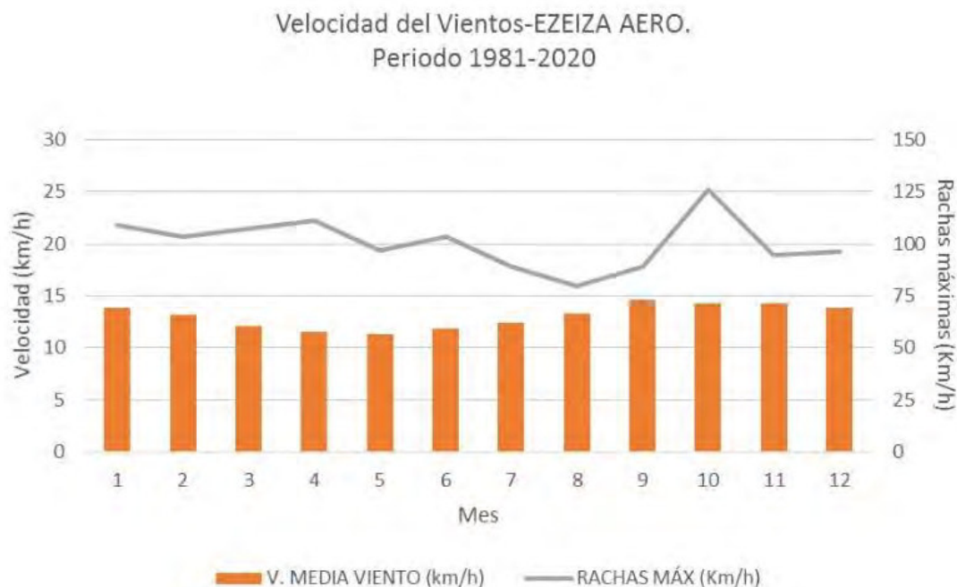
Figura 17: Media de velocidad de vientos (km/h) y rachas de viento máximas (km/h) mensuales observados en el período 1981-2020. Estación Ezeiza Aero, SMN.
