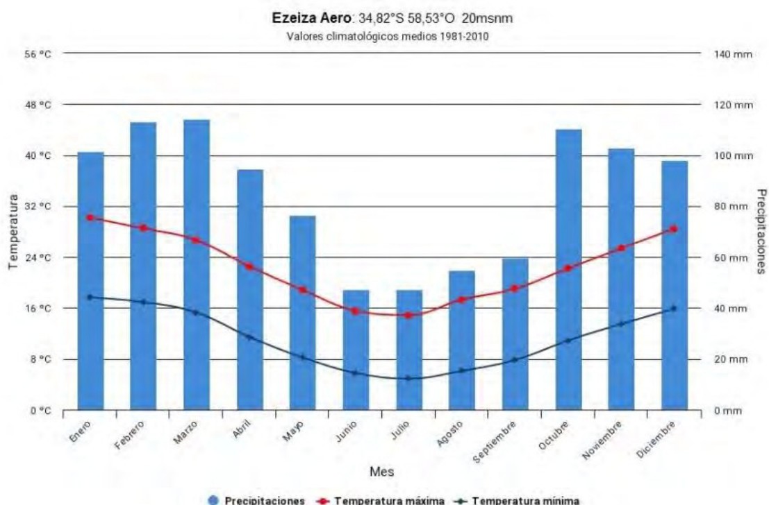
Figura 12: Climatograma extraído de las estadísticas sinópticas. Est. Met. Ezeiza Aero (SMN), período 1981–2010 24 .
